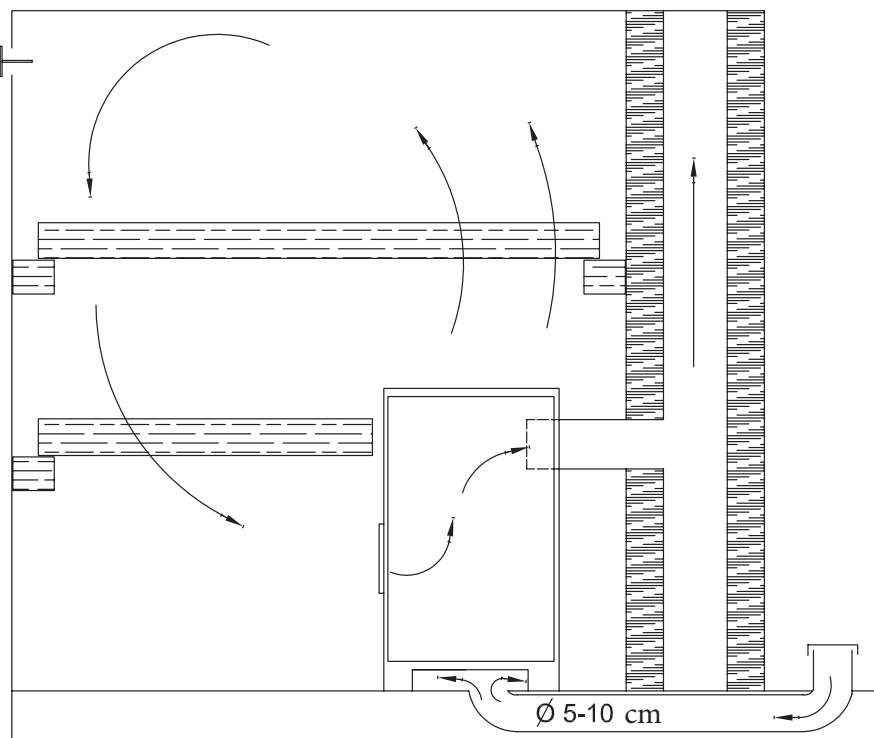
Joonis 1. Loomulik ventilatsioon Рисунок 1. Естественная вентиляция
