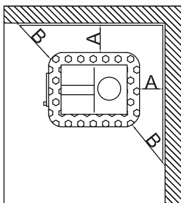
Joonis 15. Ohutud kaugused (mõõdud sentimeetrites) Рисунок 15. Безопасные расстояния (размеры в сантиметрах)
